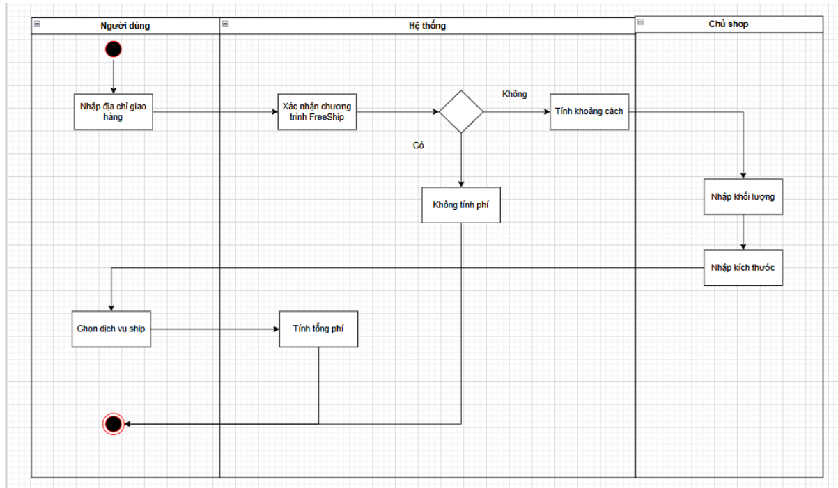
Ảnh 2. Activities diagram cho tính hóa đơn giao hàng.
