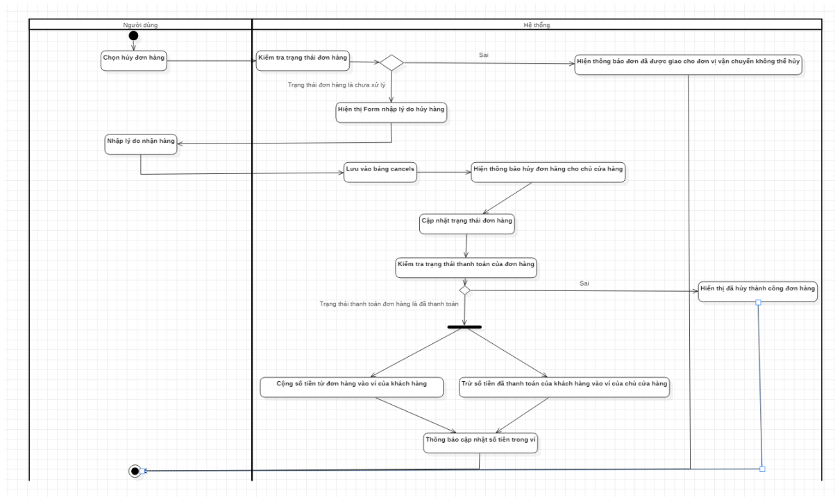
Ảnh 5. Activities diagram cho xử lý nghiệp vụ hủy đơn và hoàn tiền.
